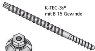
Kipp B 15 rund mit S-Mutter, verzinkt
