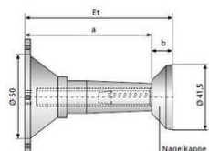
Et = Einbautiefe
