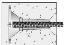
Et = Einbautiefe
