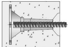
Et = Einbautiefe
