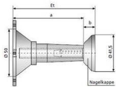
Et = Einbautiefe
